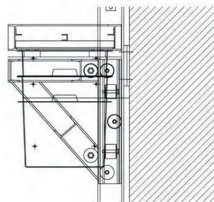
Soluzione di ancoraggio con con sistema saliscendi autoportante.
