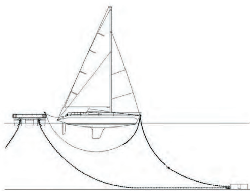
Soluzione di ancoraggio con catene e corpi morti in calcestruzzo.
